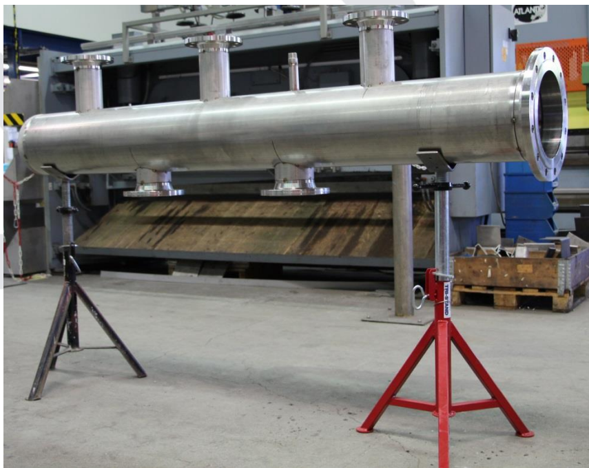
Vorfertigung eines Wasserverteilers Werkstoff 1.4571, Betriebsdruck 6 bar
